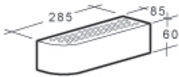
MRT (60) PYÖRISTETTY
