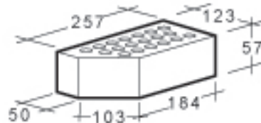
PTR VIISTETTY
