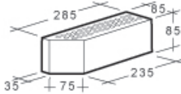
MRT (85) VIISTETTY
