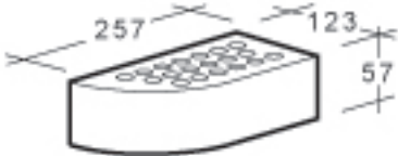
PTR PYÖRISTETTY
